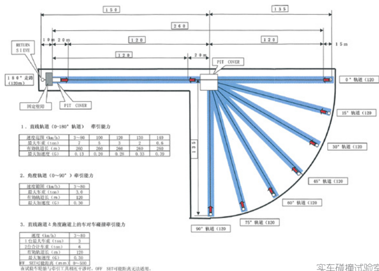
实车碰撞试验室
